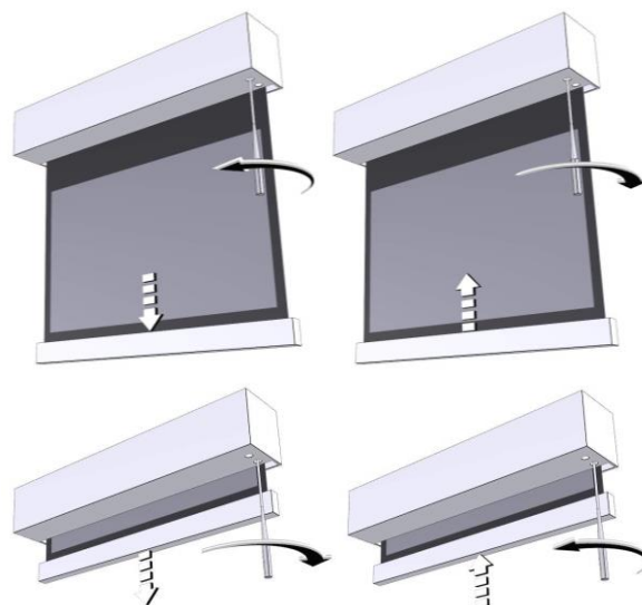
B - Motor instalada a la Derecha (standard)
