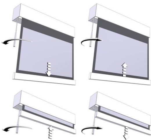
Tela se desenrolla por Delante - D
