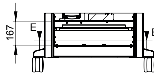
SECTION D-D SCALE 1 : 20
